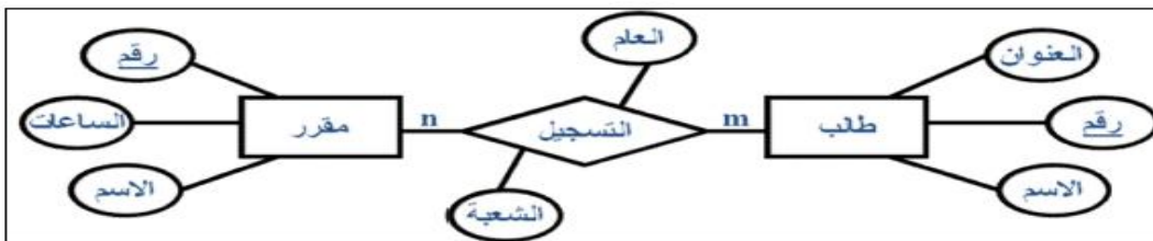
علاقة M:N كثير-إلى-كثير (many-to-many)
