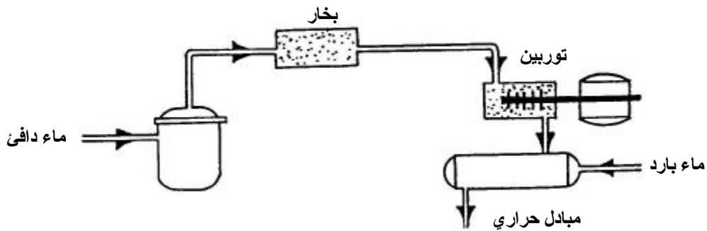
شكل (2-11): طريقة الدائرة المفتوحة لإنتاج الطاقة من حرارة مياه المحيطات
