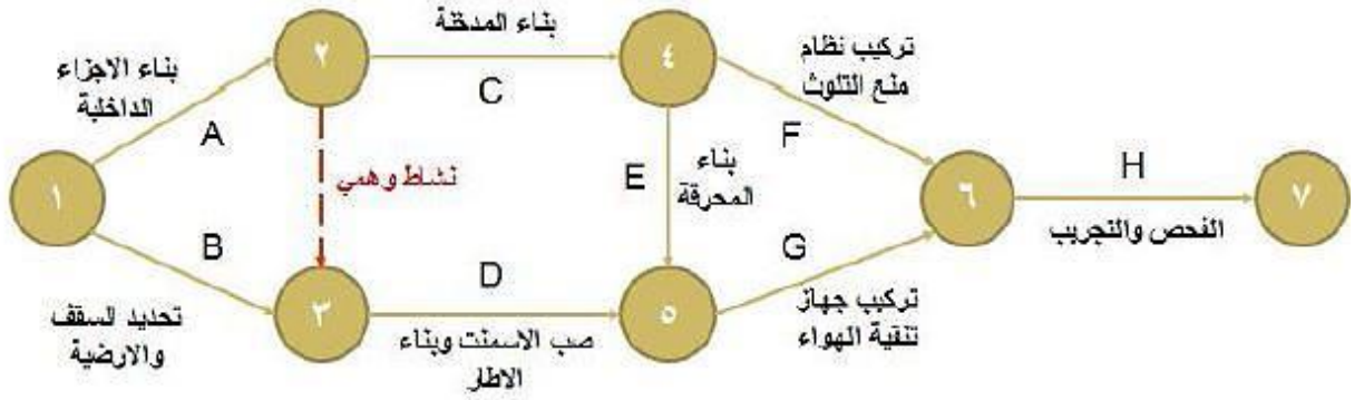
شكل ( ٥ - ٣ ) رسم شبكة مشروع محرقه ورق بإستخدام النشاط على السهم
