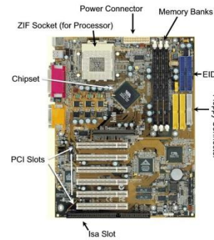
ثقوب التوسع (Expansion Slots)
