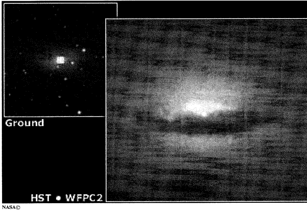
شكل (55) نجم خائس كانس يدور حول محوره ويحاط بقرص رقيق من المواد المجمعة حوله
