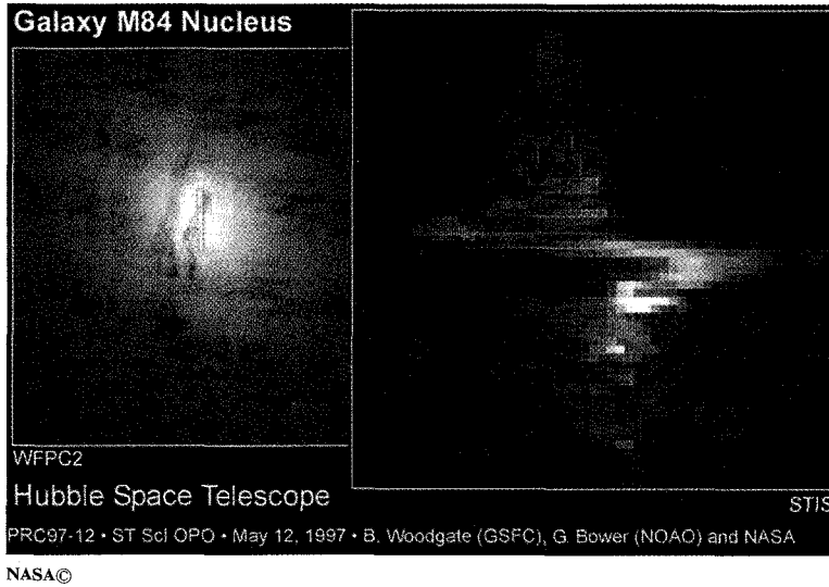
شكل (54) صورة للأثار التي تركها أحد النجوم الخانسة الكانسة (الثقوب السود) كما صورتها عدسات التليسكوب الفضائي هابل
