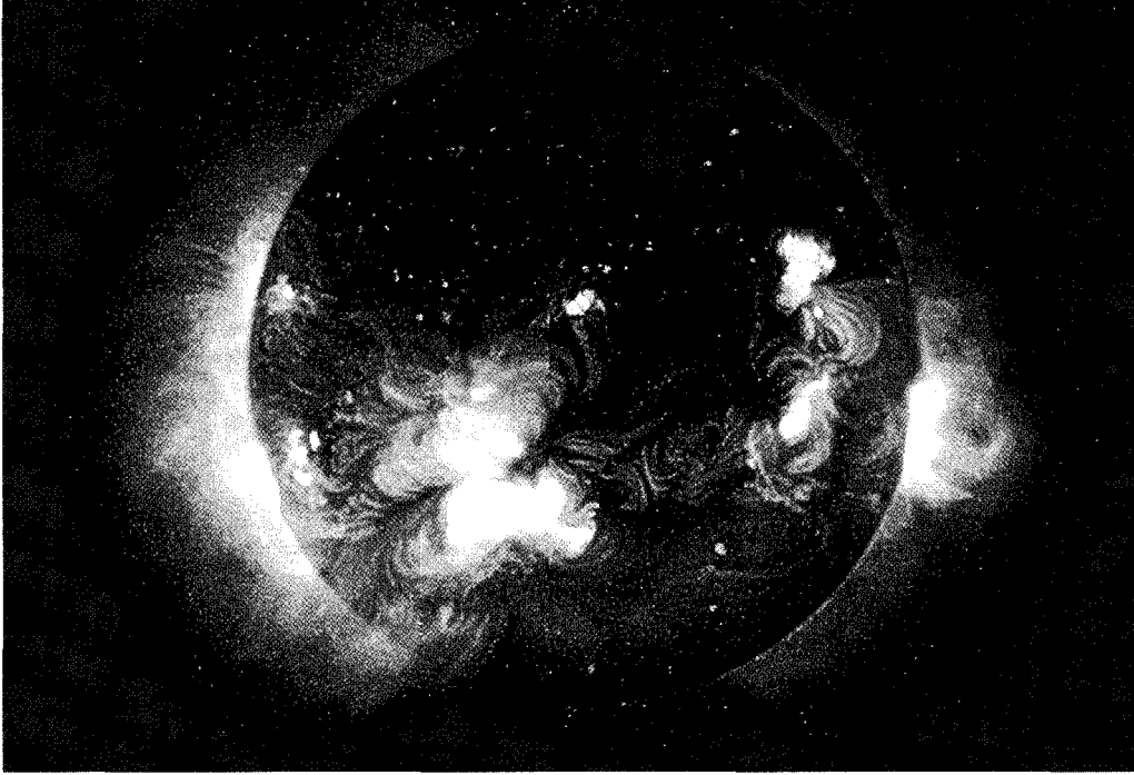
شكل (175) صورة للشمس في وقت توهجها
