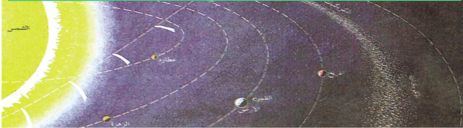
لوحة توضيحية لمدار الكويكبات
