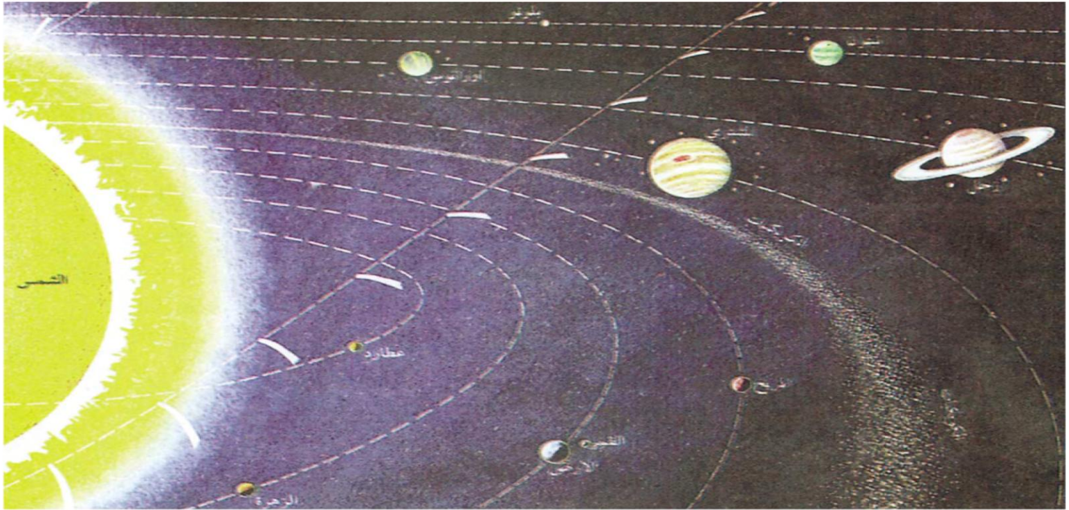
لوحة توضيحية لمدار الكويكبات
